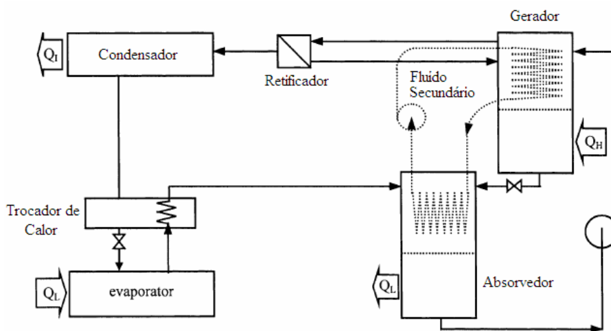
Fig. 2.4 Conceito dos ciclos GAX
