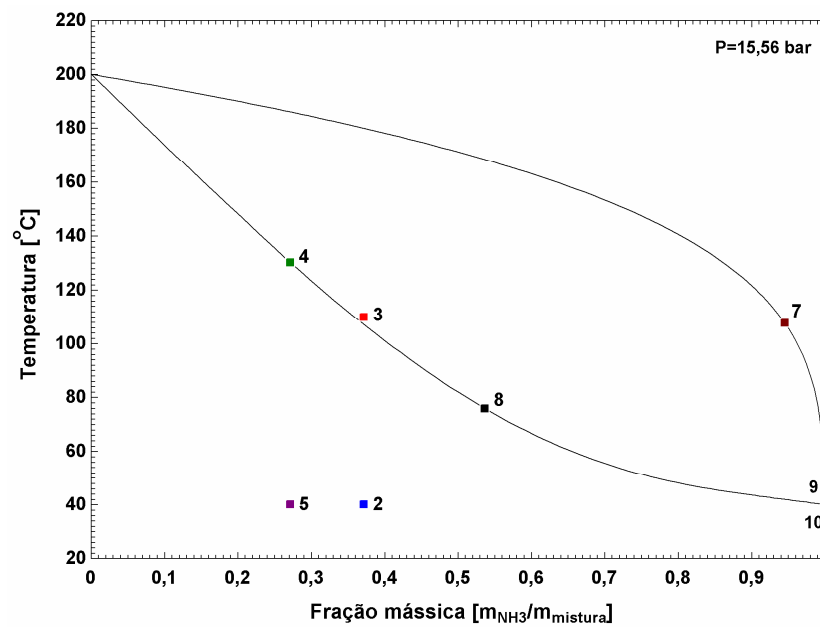
Fig. 4.18 Diagrama T - x para a pressão alta indicando os estados para o modelo variante 2
