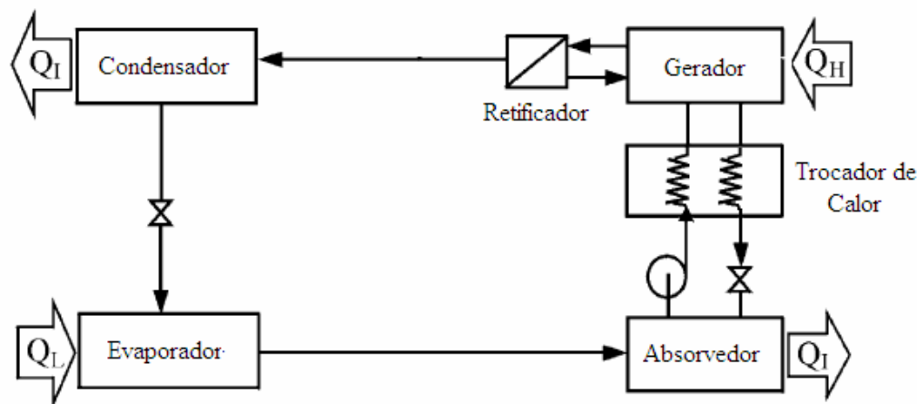
Fig. 2.2 Sistema de refrigeração por absorção de amônia
