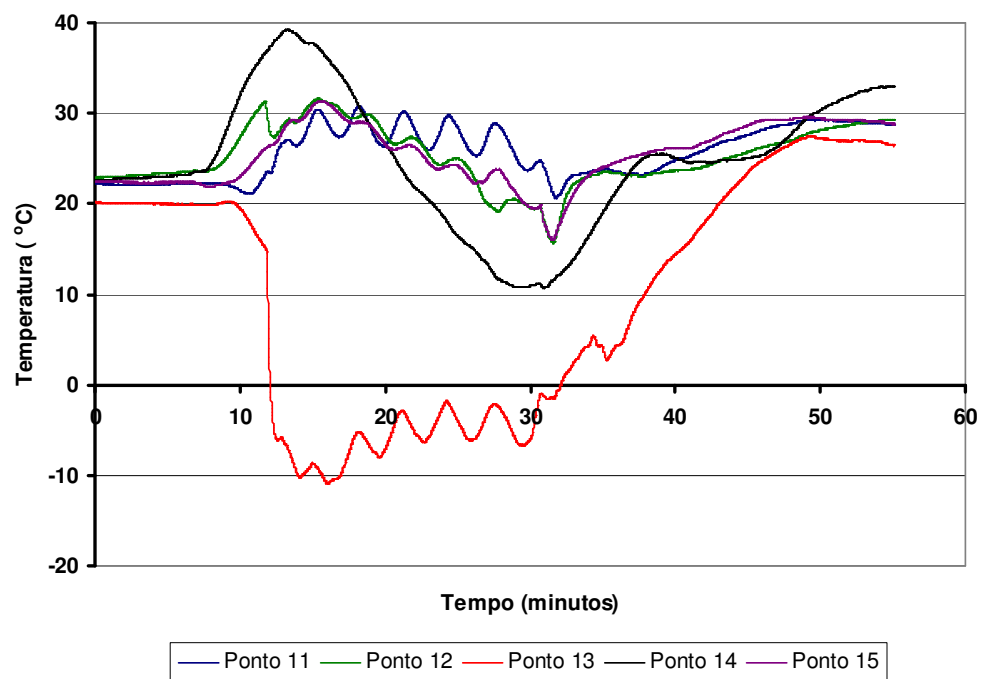
Fig. 4.35 Temperaturas nos diversos pontos do equipamento
