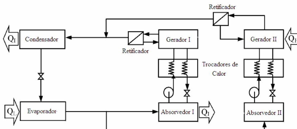
Fig. 2.3 Ciclo de refrigeração por absorção de duplo-efeito
