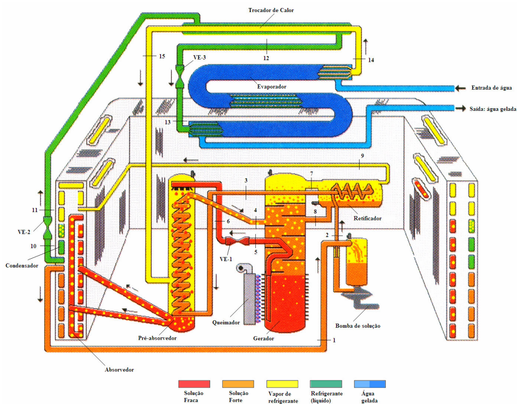
Fig. 4.20 Esquema do ciclo do equipamento
