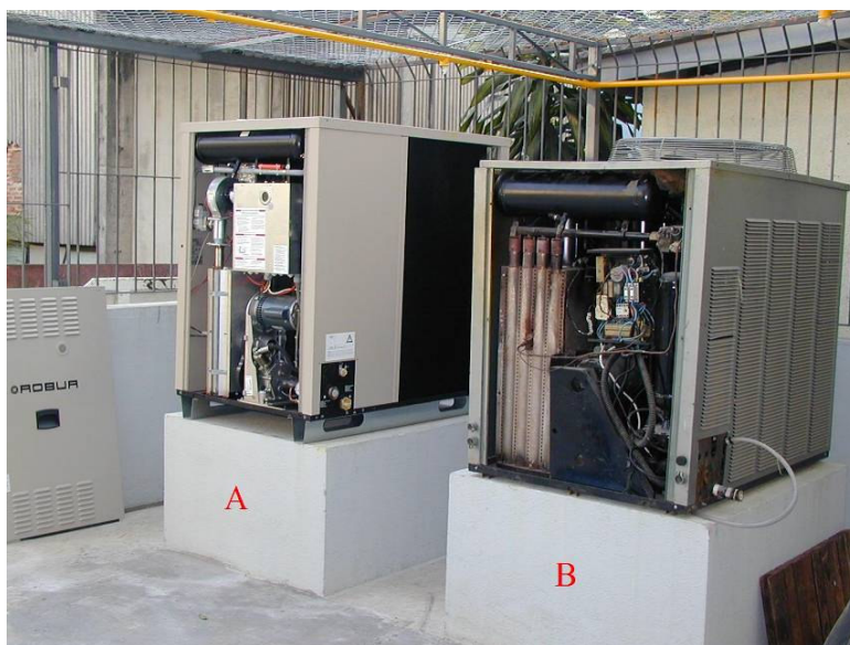
Fig. 3.1 Equipamentos utilizados nos testes (A) e na elaboração do modelo (B)
