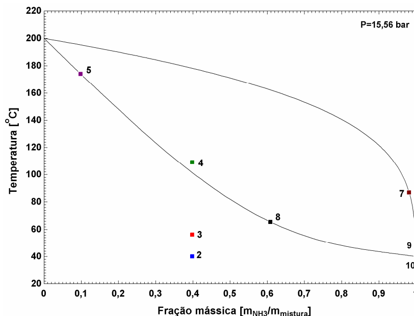
Fig. 4.29 Diagrama T-x para a pressão alta indicando os estados para o ciclo comercial
