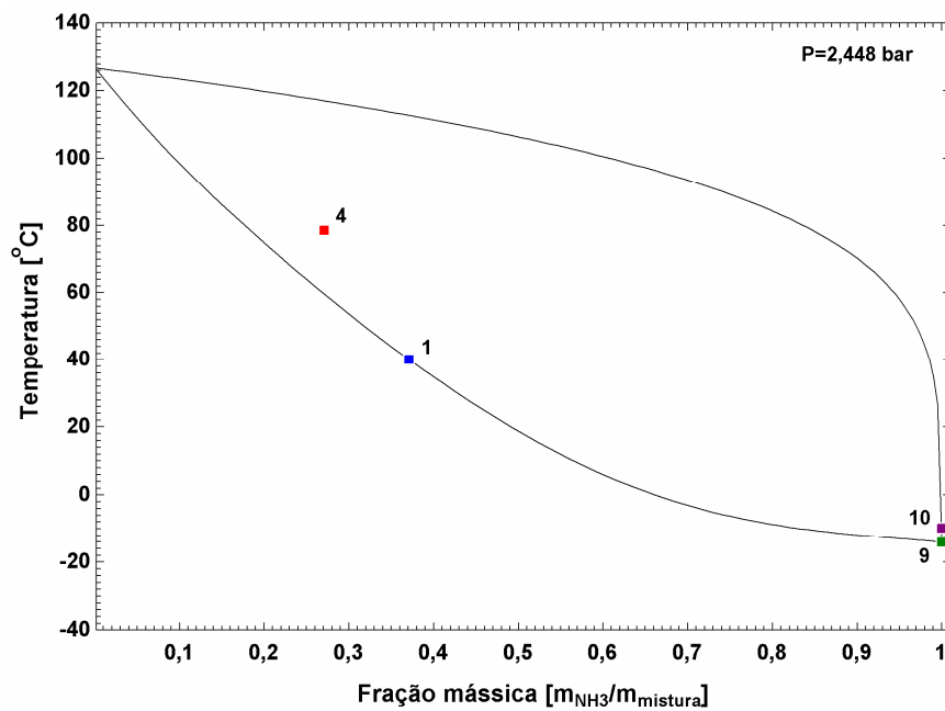
Fig. 4.13 Diagrama T-x para a pressão baixa indicando os estados para o modelo variante 1
