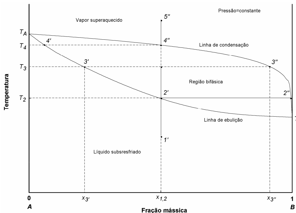
Fig. 2.1 Diagrama temperatura-fração mássica para a mistura amônia-água
