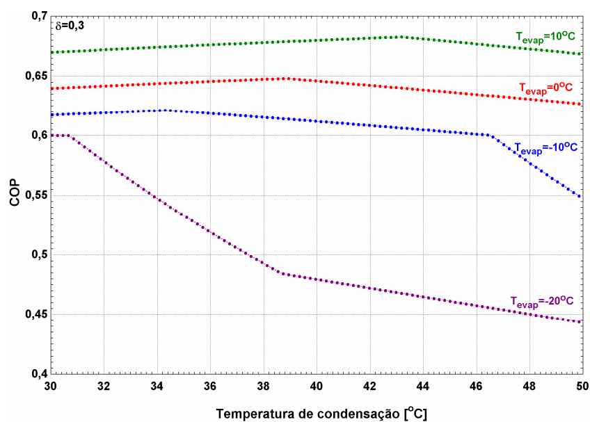
Fig. 4.30 Efeito da variação das temperaturas de condensação e evaporação no COP
