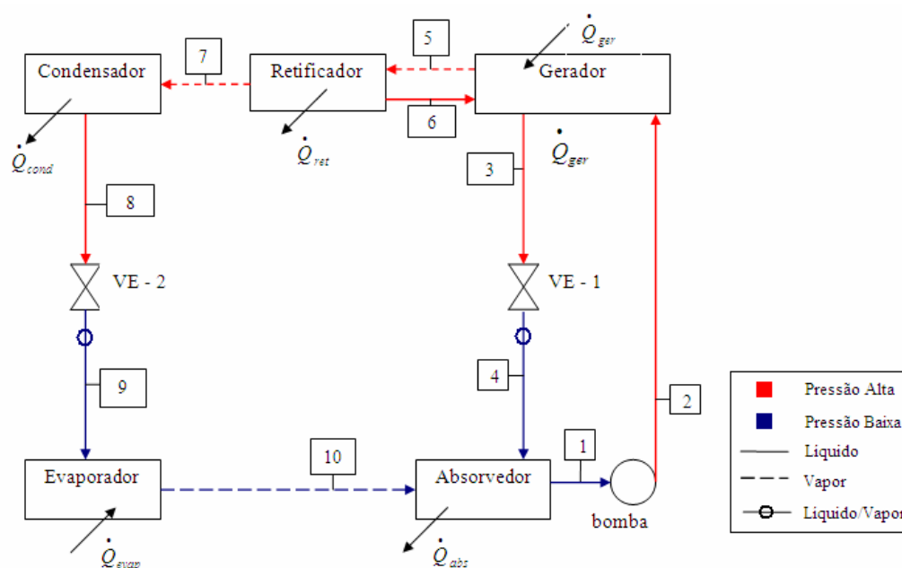
Fig. 4.10 Esquema do modelo variante 1 (ciclo com retificador)
