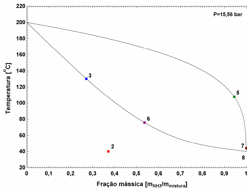
Fig. 4.14 Diagrama T-x para a pressão alta indicando os estados para o modelo variante 1
