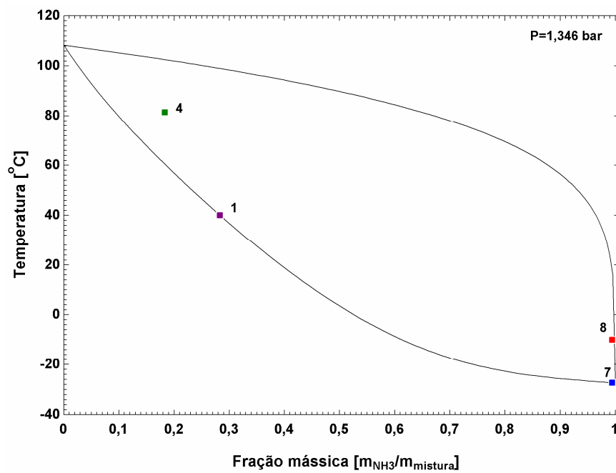
Fig. 4.8 Diagrama T-x para a pressão baixa indicando os estados para o ciclo simples
