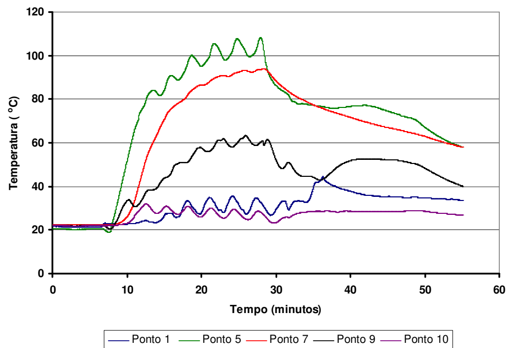
Fig. 4.34 Temperaturas observadas nos componentes do equipamento ensaiado
