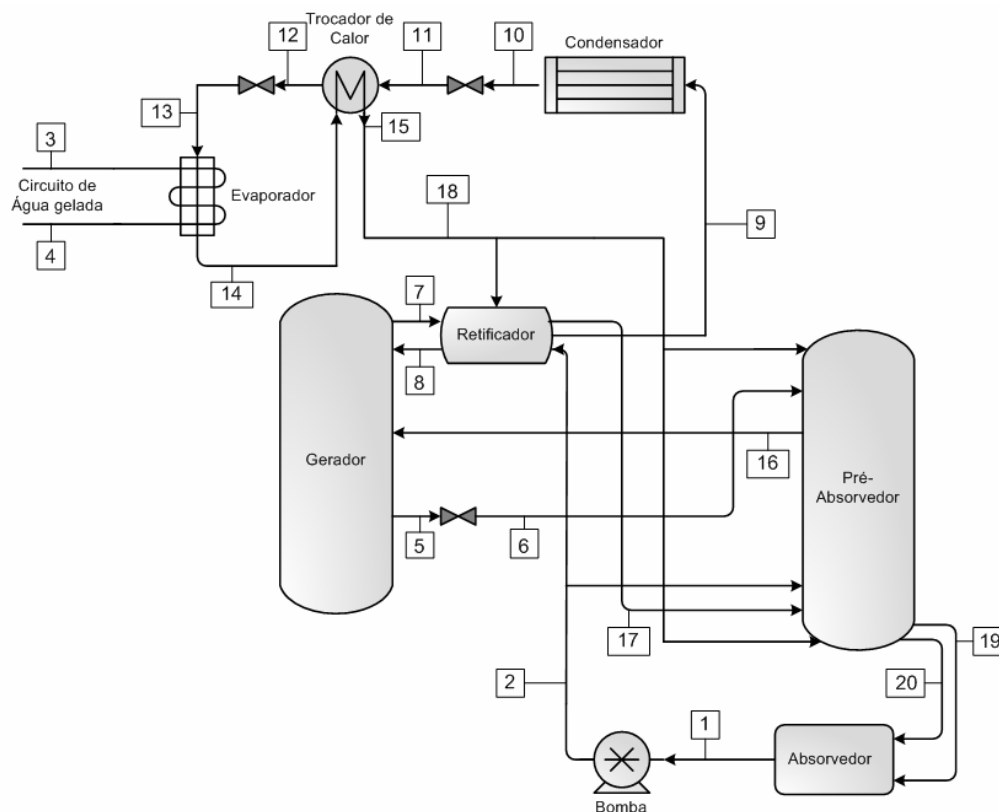
Fig. 4.33 Esquema do equipamento utilizado nos ensaios
