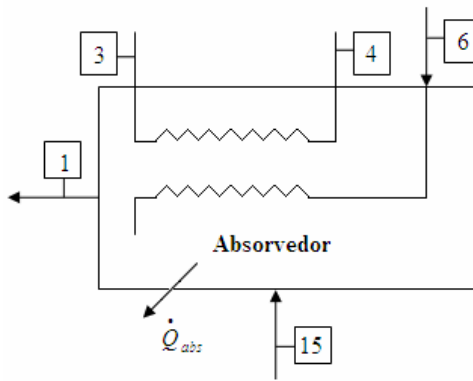
Fig. 4.25 Esquema do absorvedor
