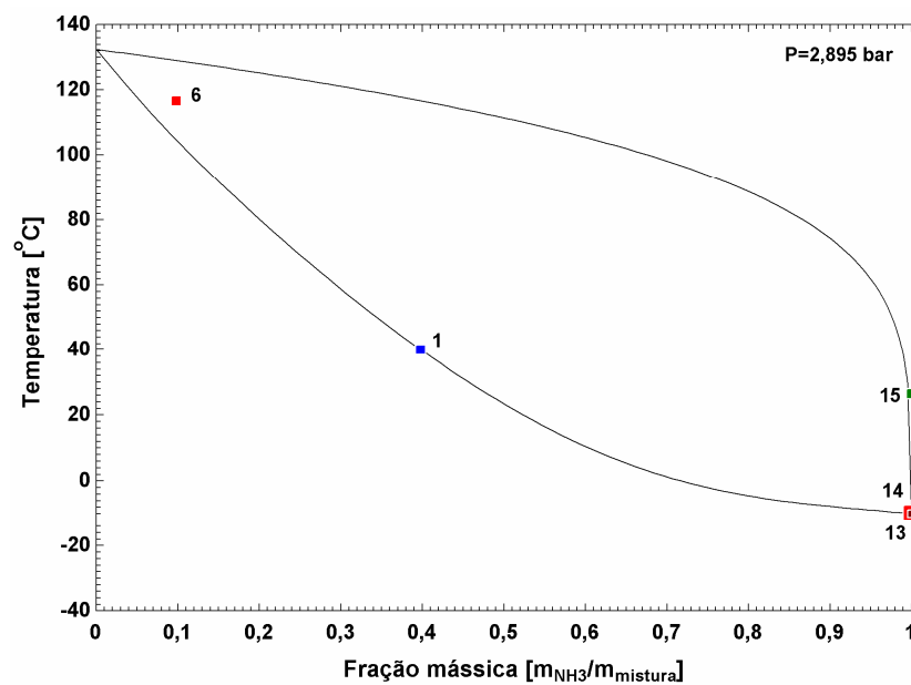
Fig. 4.27 Diagrama T - x para a pressão baixa indicando os estados para o ciclo comercial
