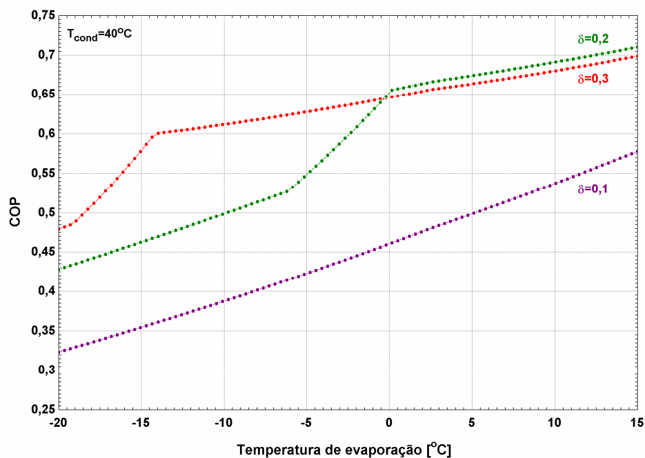
Fig. 4.32 Efeito da variação da temperatura de evaporação no COP
