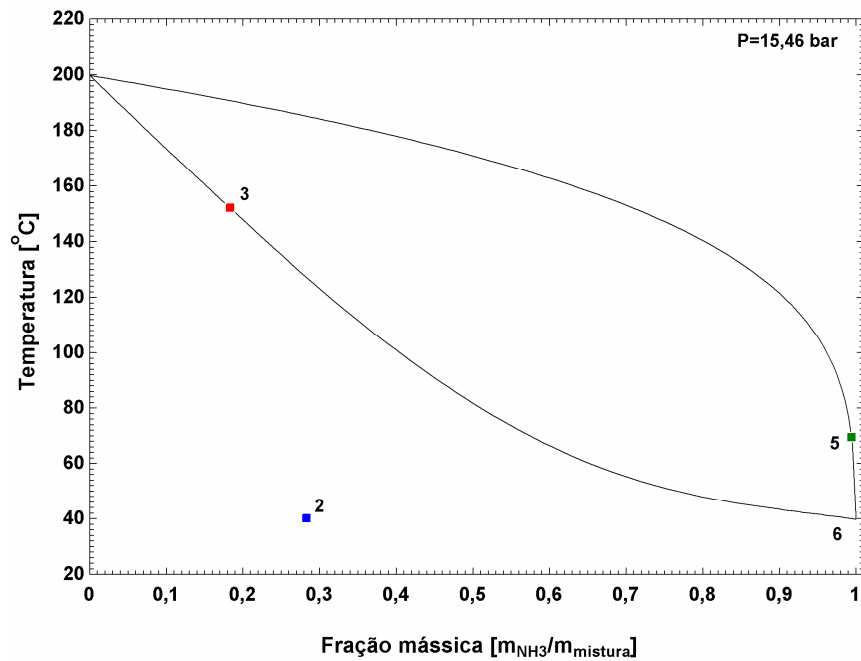
Fig. 4.9 Diagrama T-x para a pressão alta indicando os estados para o ciclo simples
