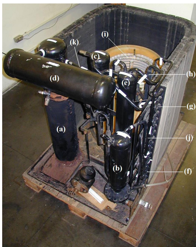
Fig. 4.19 Equipamento estudado com a identificação de seus componentes
