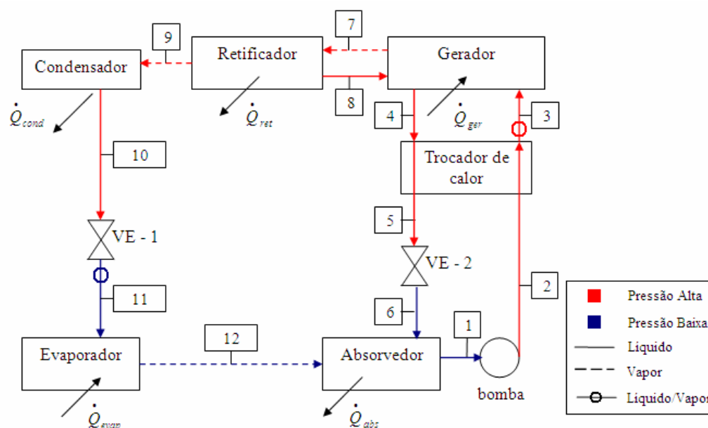
Fig. 4.15 Esquema do modelo variante 2
