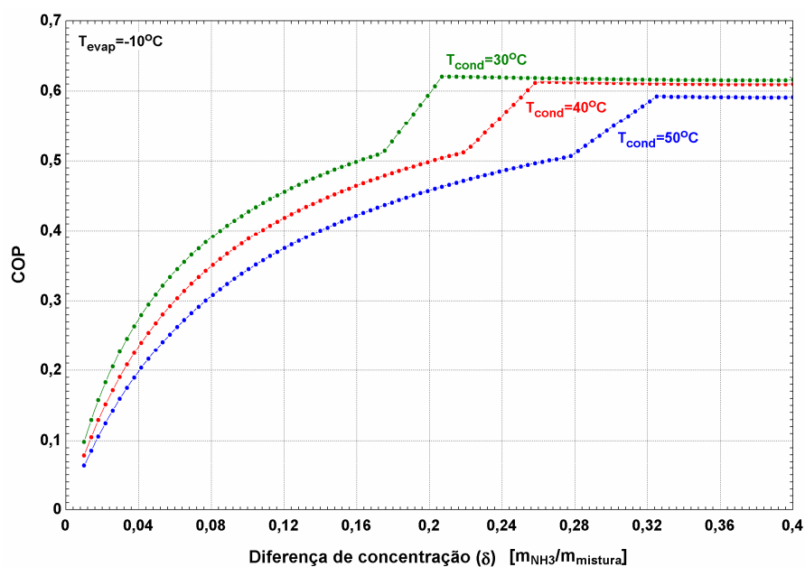
Fig. 4.31 Efeito da variação da diferença de concentração no COP
