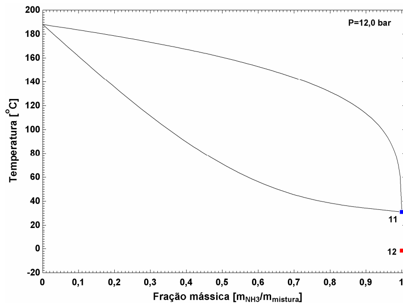
Fig. 4.28 Diagrama T - x para a pressão intermediária indicando os estados para o ciclo comercial
