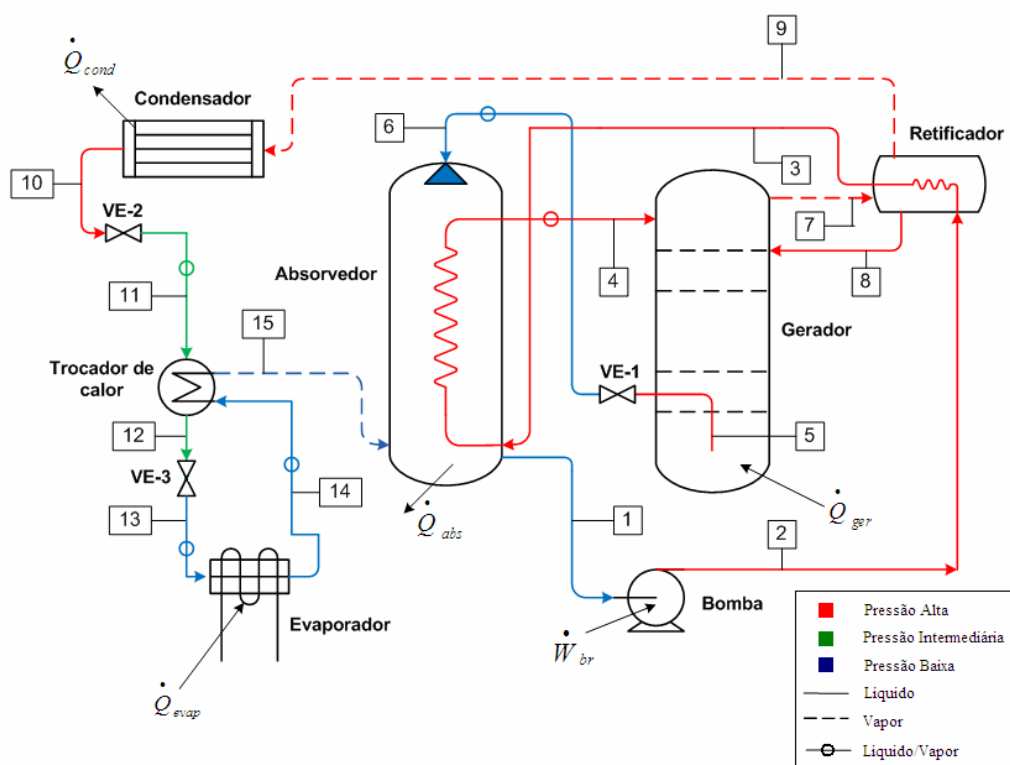
Fig. 4.21 Modelo do ciclo comercial
