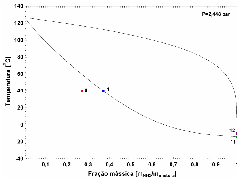
Fig. 4.17 Diagrama T - x para a pressão baixa indicando os estados para o modelo variante 2
